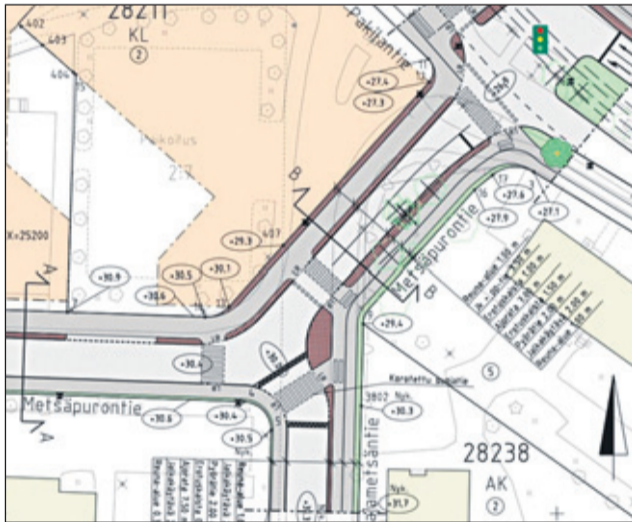
Ote rakennusviraston lähettämästä Metsäpurontien katusuunnitelmasta.
